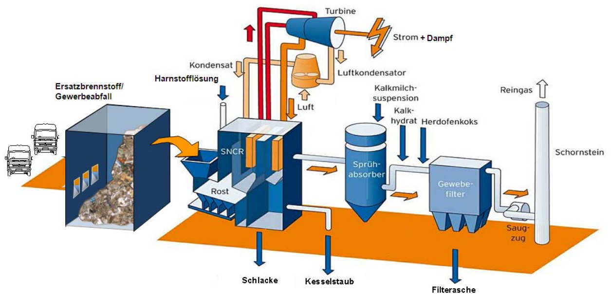
Abbildung 1: Vereinfachtes Verfahrensfliessbild
